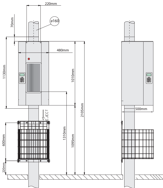
Måttangivelser station och montering
